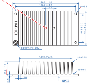
外形図(2D)
